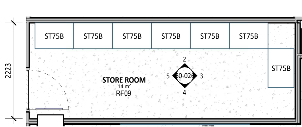
1 PLAN DETAIL 1 : 50
